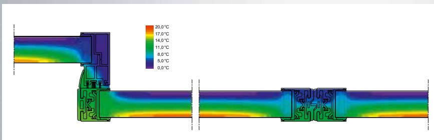
Immagine termica di porta scorrevole a due ante con anta fissa
